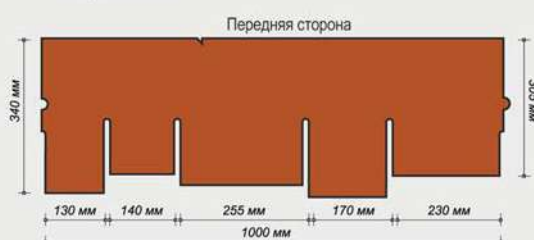
Размеры Ambient
